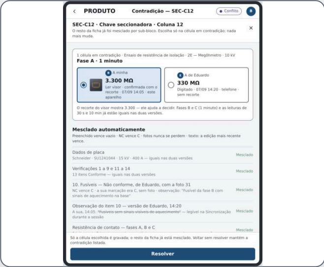
Contradição. Uma célula por linha, o recorte de quem leu pelo visor, dois botões de 56 px.
